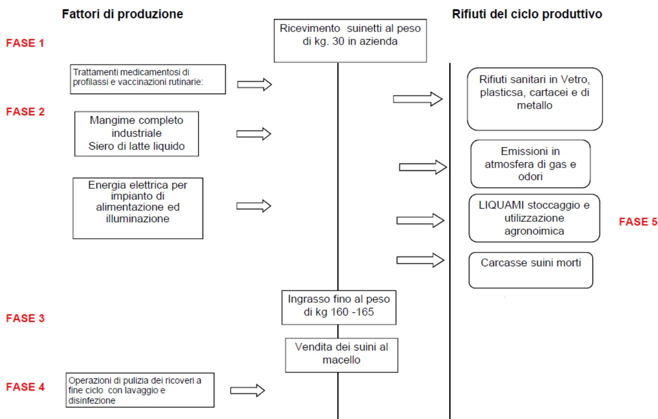
Fig. 27. Schema del ciclo produttivo dell'allevamento avicolo
