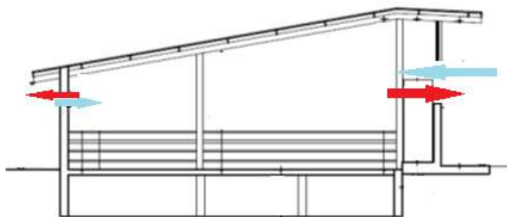
Fig.26. Schema della ventilazione naturale
