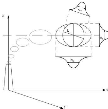
Fig.53 Schema per un modello a puff con indicazione dei coefficienti di dispersione relativi al puff k
