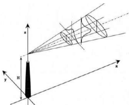
Fig.51 Rappresentazione tridimensionale dell'emissione secondo un modello gaussiano
