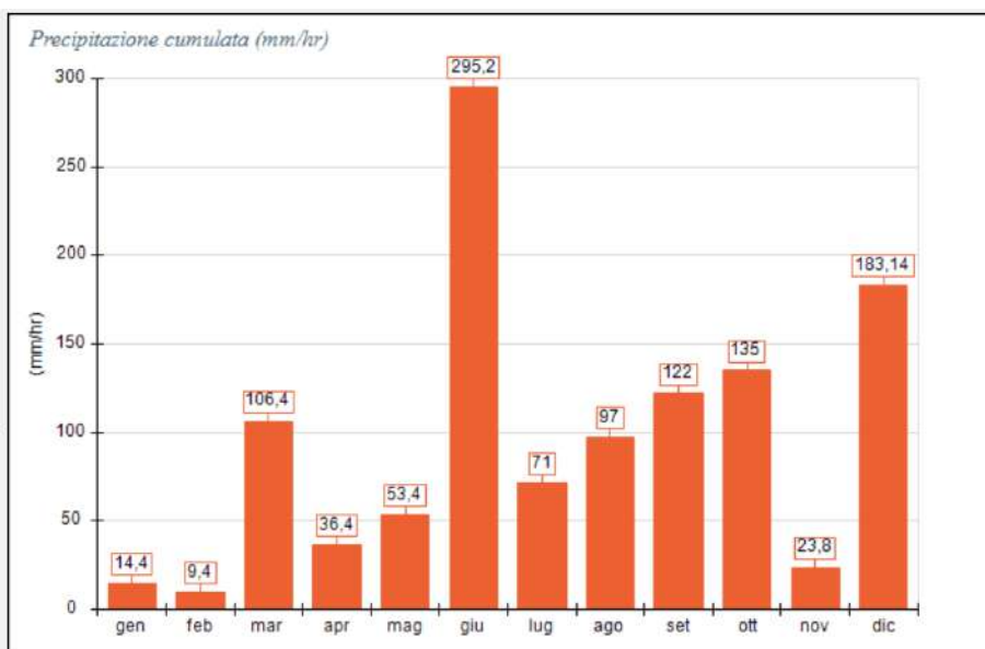
Fig. 64 Dati delle precipitazioni del 2020 presenti in MMS CALMET
