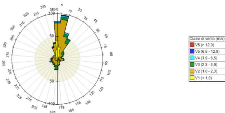
Fig.64 Rappresentazione della rosa dei venti in Inverno
