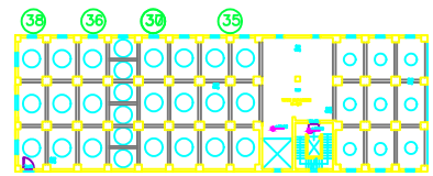
MAGAZZINO FARINE PIANA PIANO SETTIMO a quota ml. + 39,62
