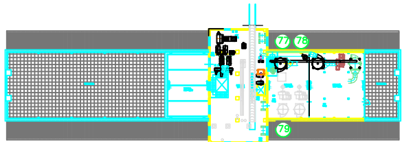
SILOS GRANO PIANA PIANO SESTO a quota ml. + 29,28 H = ml. 5,80
