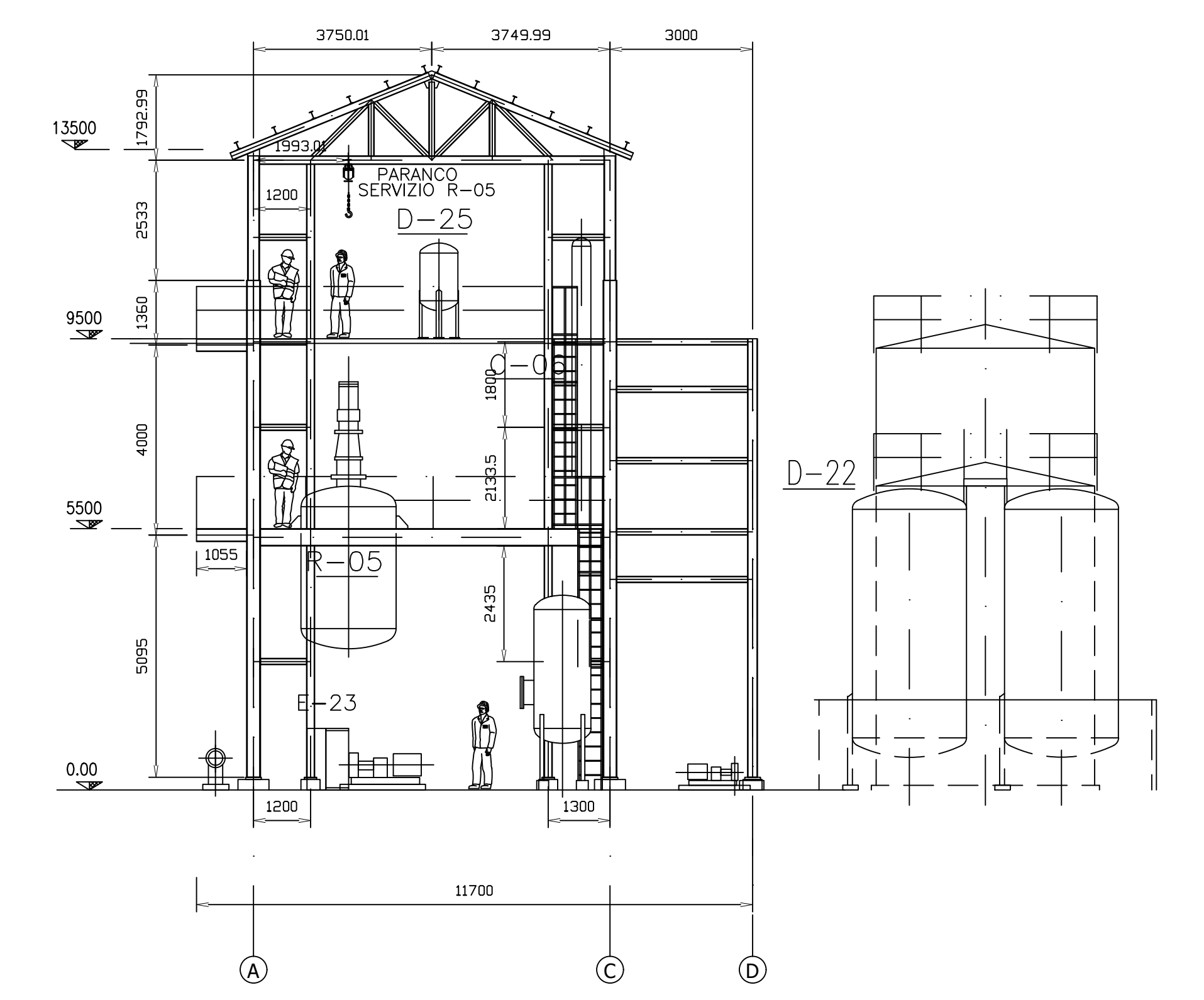
VISTA TRASVERSALE SCALA 1:100
