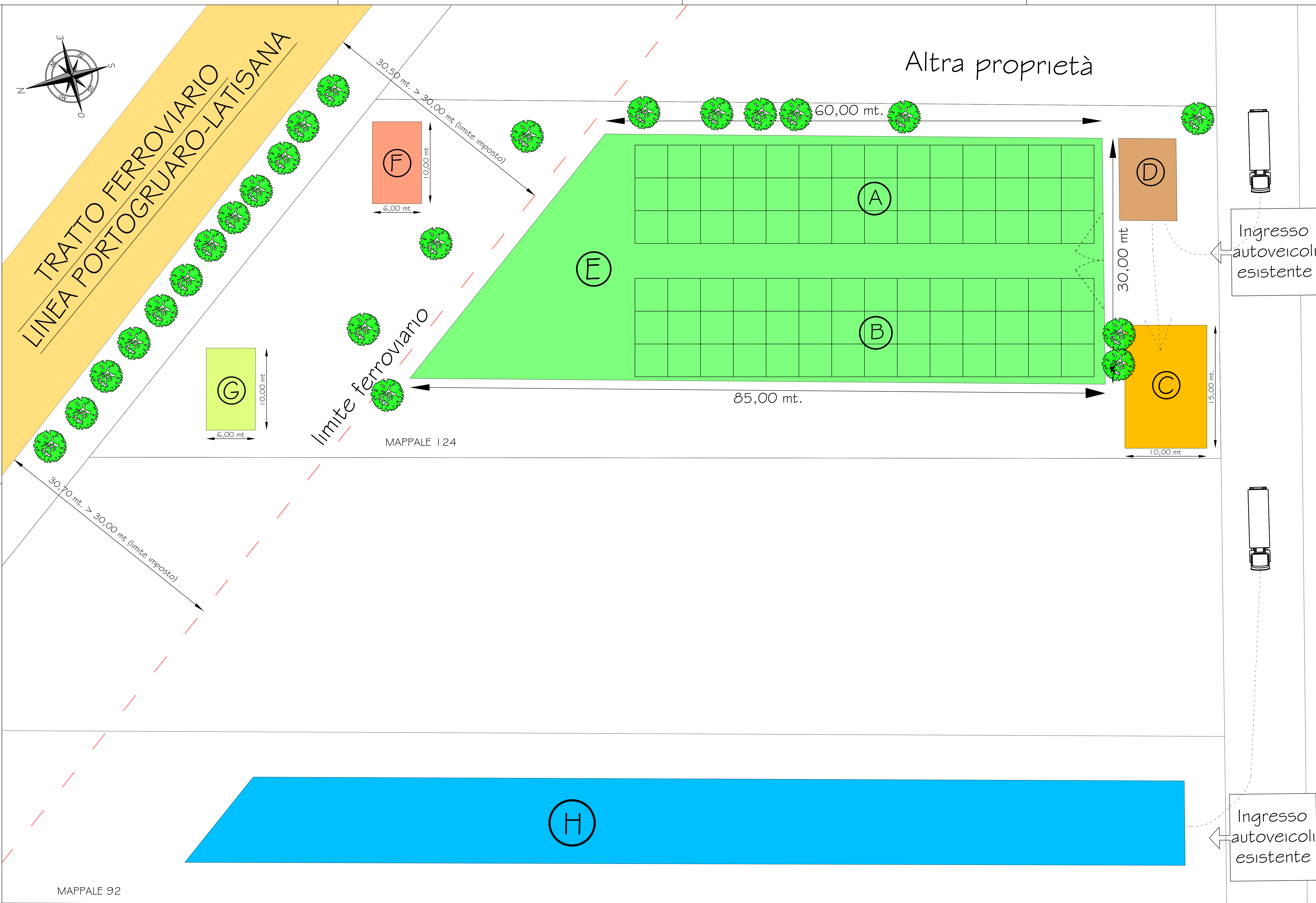
PLANIMETRIA Scala 1:200
