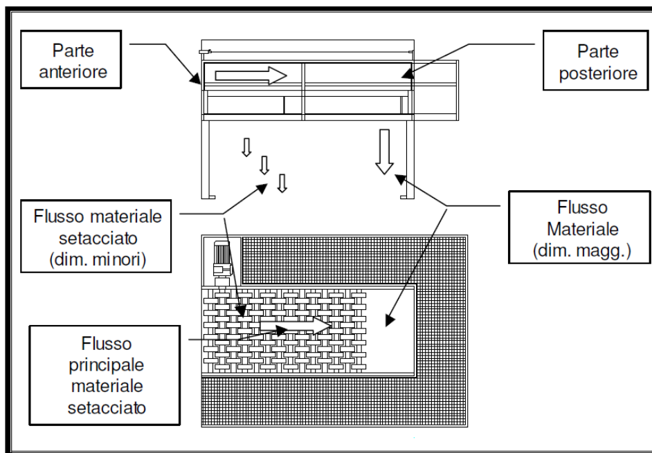
Figura 10 – Flusso del materiale attraverso il vaglio dinamico
