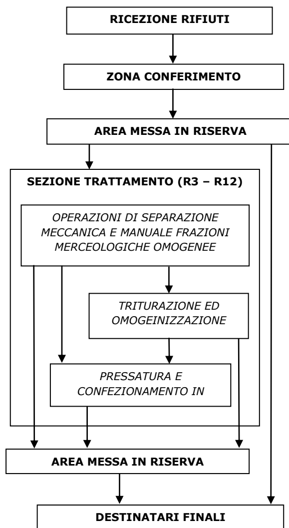
Figura 12 – Layout processo di trattamento rifiuti plastici
