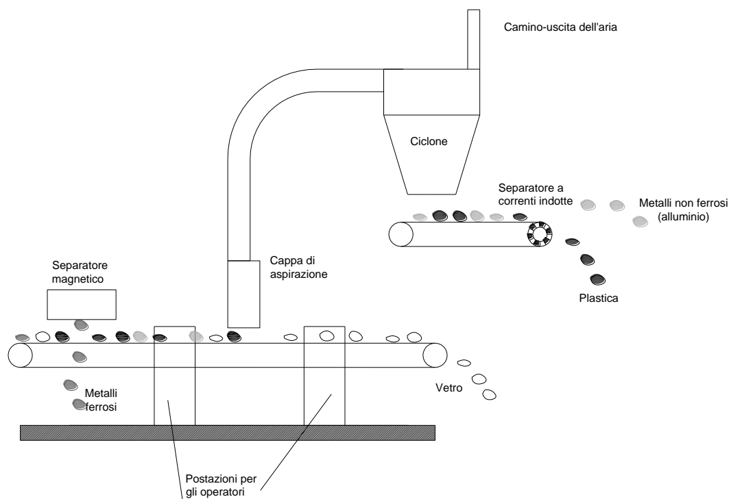
Figura 8 – Schema di funzionamento della linea di selezione VPL.
