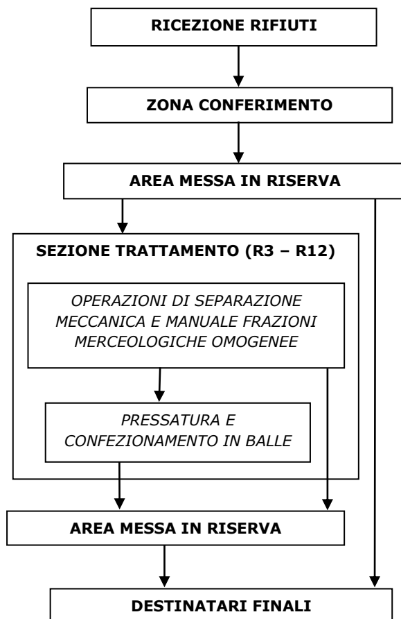
Figura 11 – Layout processo di trattamento rifiuti cartacei
