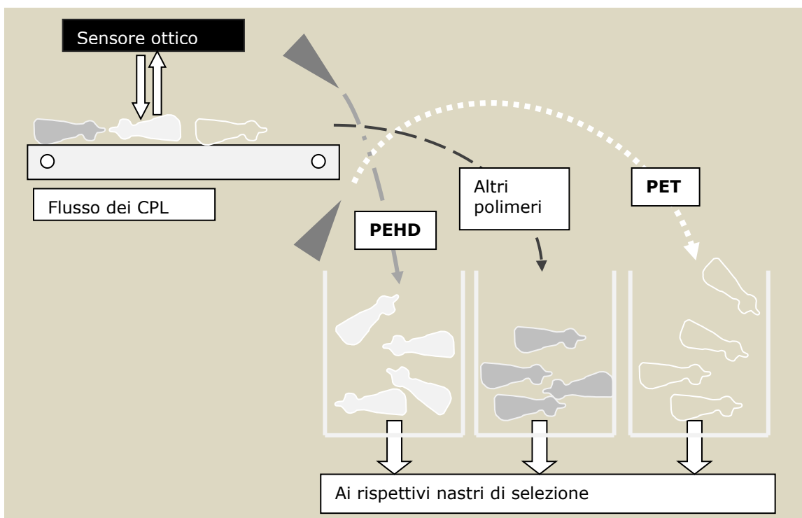
Figura 9 – Schema di funzionamento separatore ottico.
