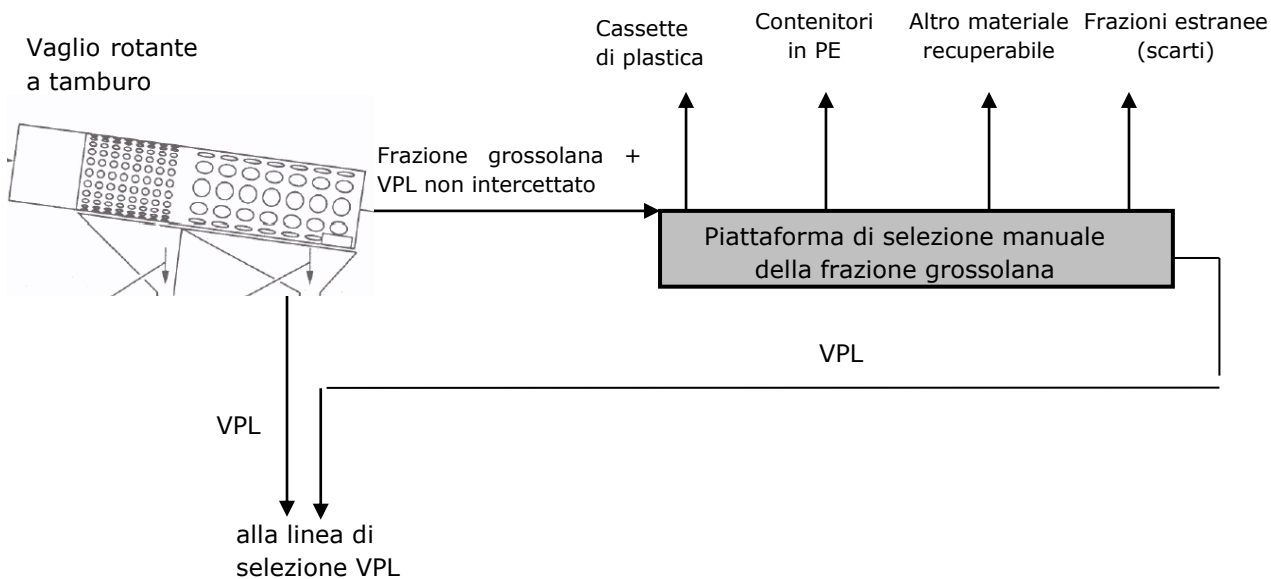
Figura 7 – Piattaforma di selezione manuale sopravaglio.
